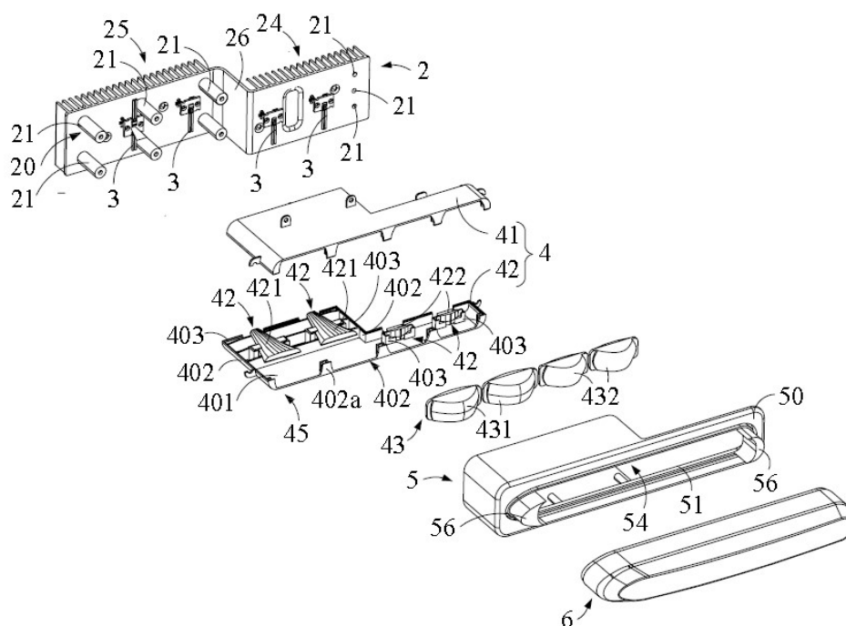
圖九、本公司導光式的遠、近燈架構
